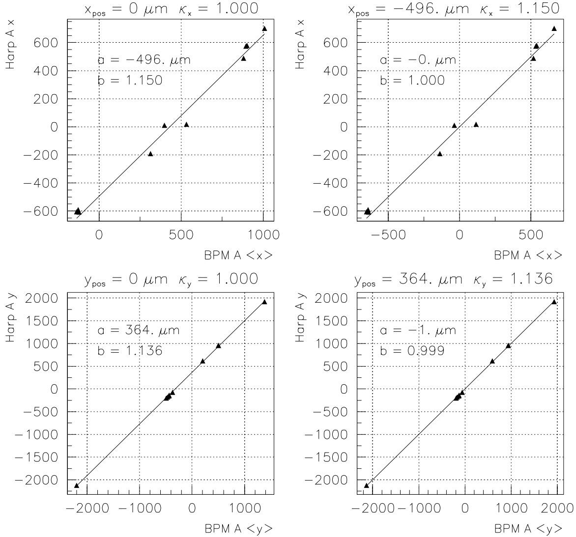
FIG. 3.1 – Calibration du BPM A : données du profileur A ( \mu\text{m} ) en fonction de la moyenne sur un run des données du BPM A ( \mu\text{m} ). À gauche avec x_{\text{pos}} = y_{\text{pos}} = 0 et \kappa_x = \kappa_y = 1 ; à droite avec des coefficients optimisés.
