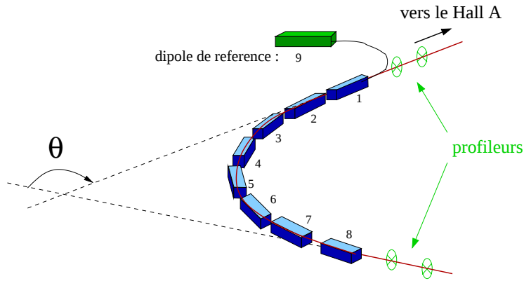
FIG. 2.8 – Principe de mesure de la méthode Arc [57].
