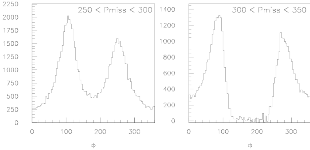
FIG. 5.11 – Distribution de l'angle hors-plan \Phi pour la cinématique 24.
