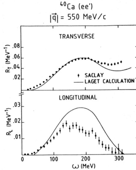
FIG. 5 – Réponses longitudinale et transverse sur le ^{40}\text{Ca} [9]. Le trait plein comprend un modèle de particules indépendantes et la contribution des courants d'échange mésoniques et de la production de \pi .
