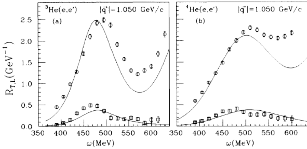
FIG. 6 – Réponses longitudinale (carrés ouverts) et transverse (cercles ouverts) sur l' ^3\text{He} et l' ^4\text{He} [16].
