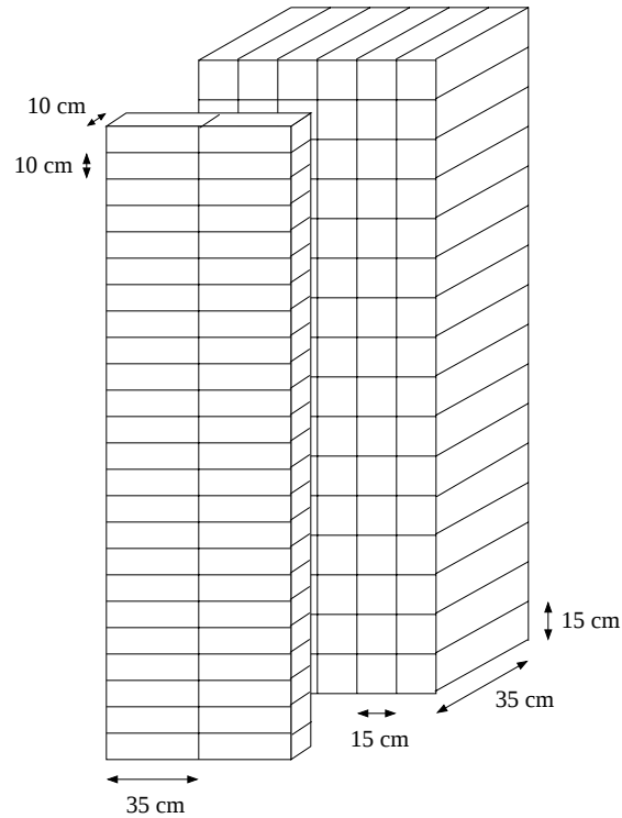
FIG. 2.19 – Géométrie des calorimètres électromagnétiques : au premier plan, le détecteur de pieds de gerbes ; en arrière plan, le détecteur de gerbes
