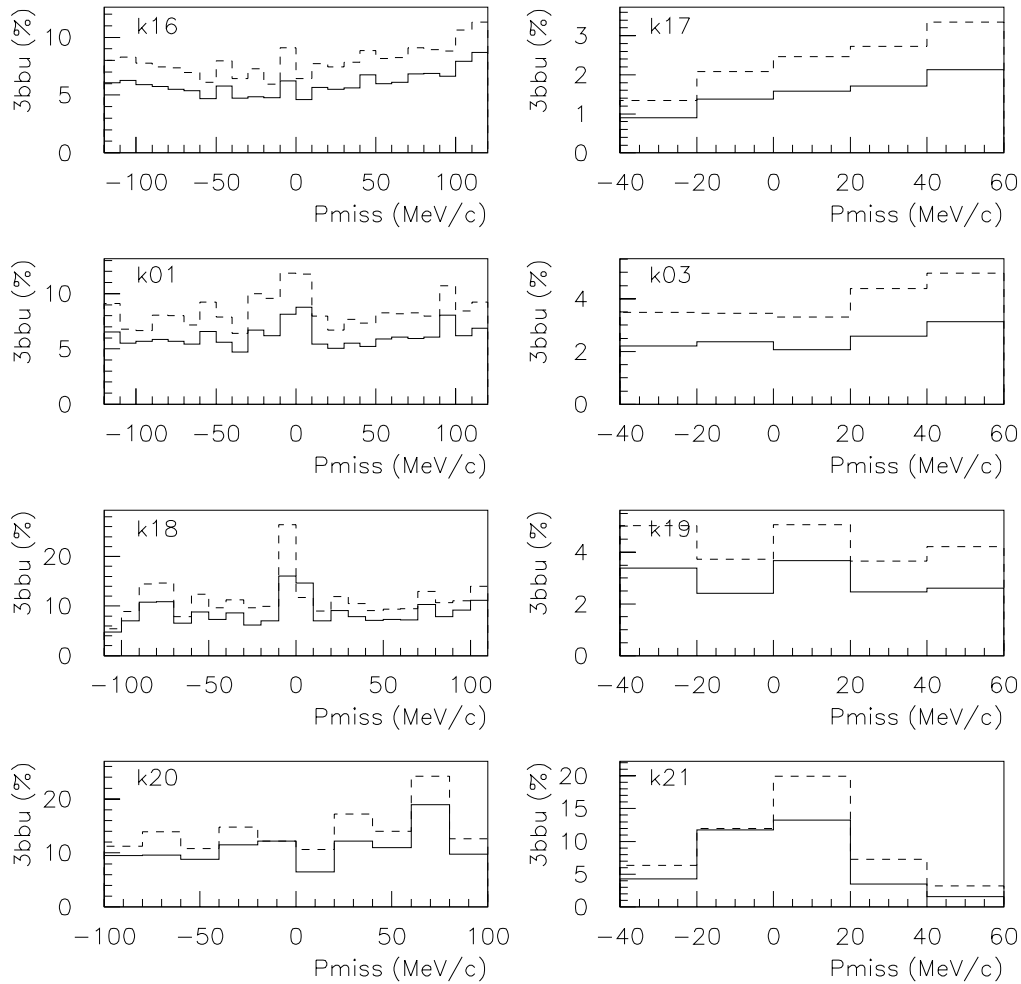
FIG. 6.8 – Proportion d'événements de 3-bbu issus de la queue de résolution inclus dans le canal en énergie manquante 0 < E_{miss} < 7.7 MeV par rapport au nombre total d'événements dans cet intervalle (cinématiques à p_{miss} = 0 MeV/c) : les traits pleins correspondent aux résultats avec le modèle indépendant, les tirets aux résultats avec le modèle onde plane.
