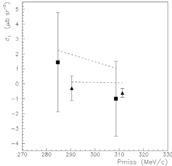
FIG. E.1 – Fonctions de réponses longitudinales pour les cinématiques à p_{\text{miss}} = -300 MeV/c : à Q^2 = 0.8 \text{ GeV}^2 (carrés noirs) et Q^2 = 1.5 \text{ GeV}^2 (triangles noirs). Les résultats ponctuels sont comparés aux prédictions théoriques du modèle en ondes planes de De Forest/Salme (tirets) calculées au point cinématique défini par les valeurs moyennes de \omega , q et p_{\text{miss}} .
