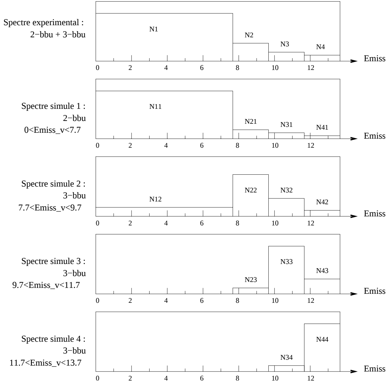
FIG. 6.1 – Schéma de la décomposition des spectres en énergie manquante E_{\text{miss}} selon le processus concerné : définition des notations pour les nombres d'événements.
