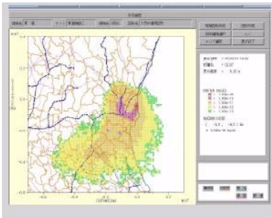
WSPEEDI
