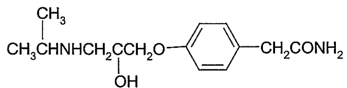
Atenolol
