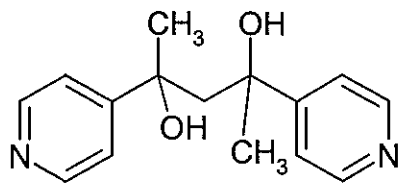
2,3-di(4-pyridyl)-2,3-butanediol
