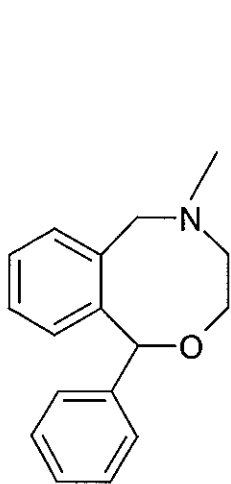
Nepofam
