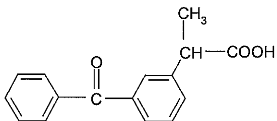
Ketoprofen
