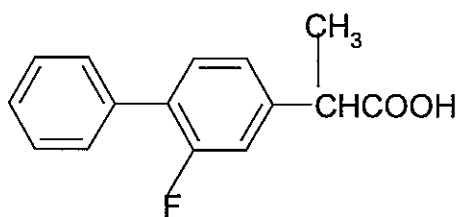
Flurbiprofen
