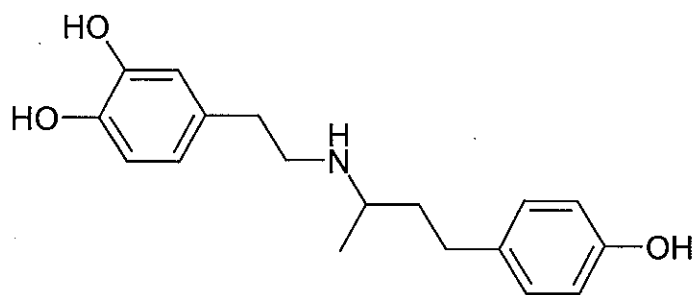
Dobutamine
