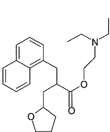
Nafrotyl
