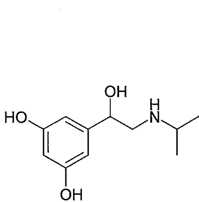
Metaproterenol
