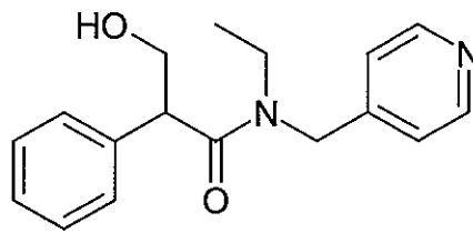
Tropicamide
