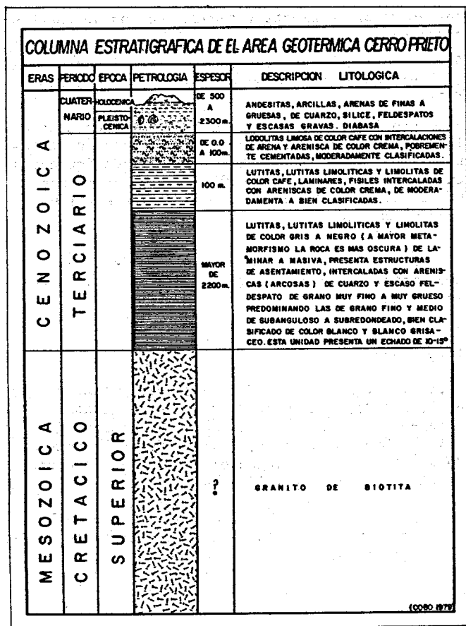
Figura 1. Columna estratigráfica del area de Cerro Prieto.
