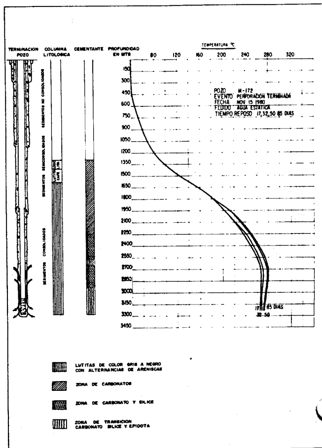
Figura 9. Registros de temperatura del pozo M-172 después de su terminación.
