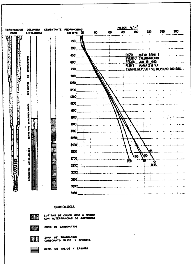
Figura 8. Registros de presión del pozo Nuevo León 1 durante su calentamiento.
