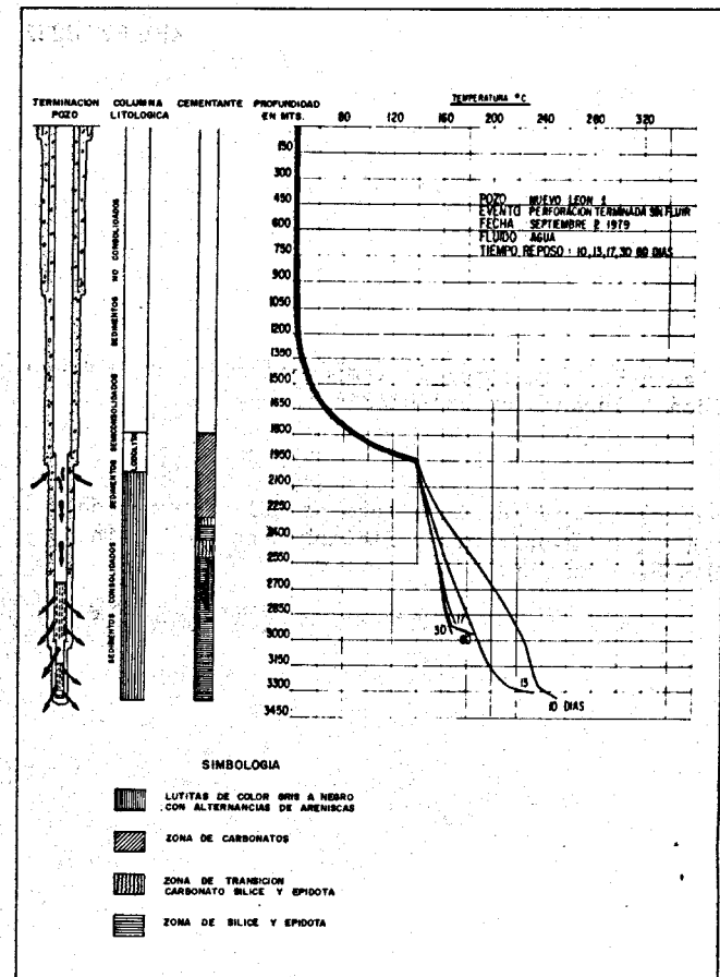
Figura 3. Registros de temperatura del pozo Nuevo León 1 después de eliminar el lodo de perforación.
