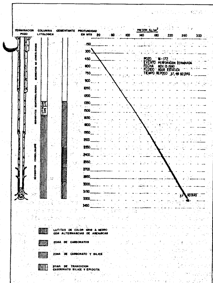
Figura 10. Registros de presión del pozo M-172 después de su terminación.
