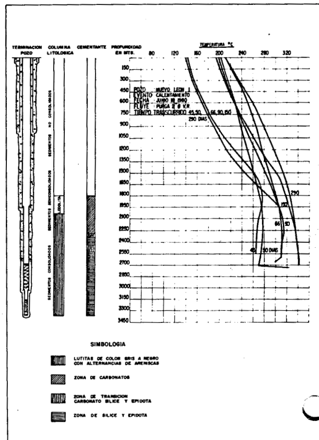
Figura 5. Registros de temperatura del pozo Nuevo León 1 durante su calentamiento.
