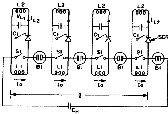
Fig. IX-9. Notch circuit.
