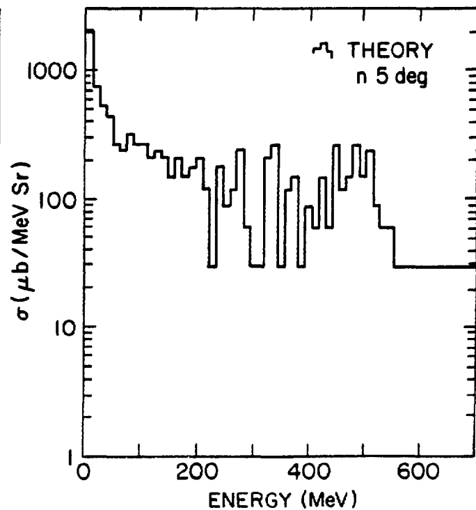
Al + piplus 800 MeV/c
