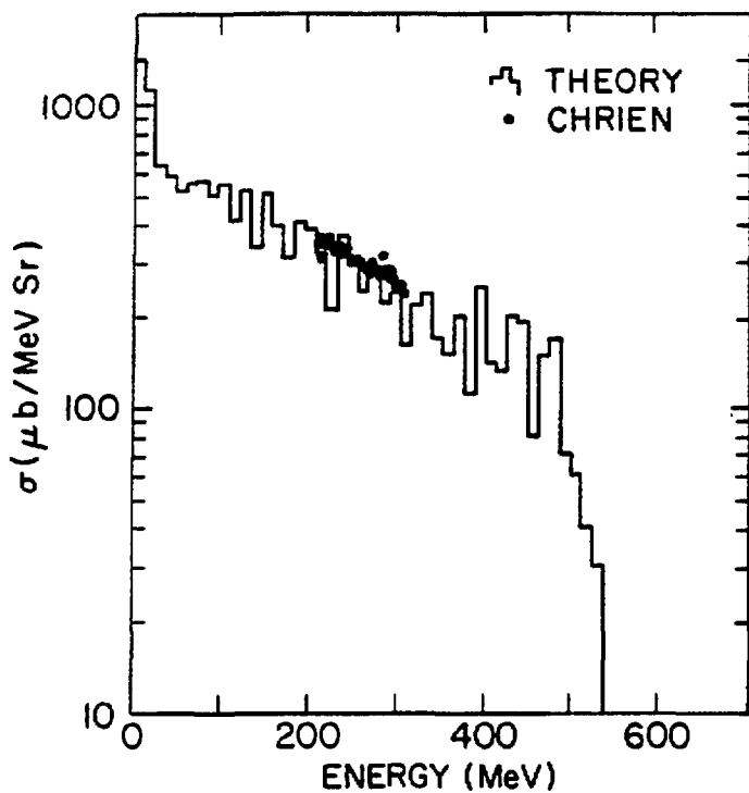
Al + piplus 800 MeV/c
