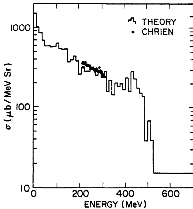
Al + piplus 800 MeV/c
