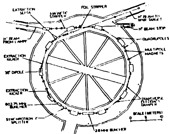
Fig. 5. PSR layout.
