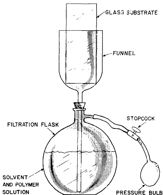
Fig. VI-4. Film-casting apparatus.
