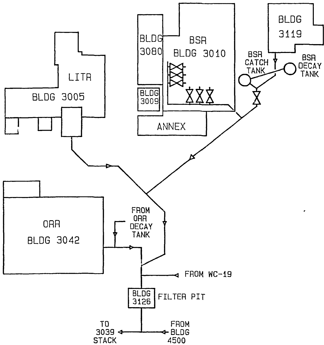
Fig. 7.2. BSR-ORR normal off-gas, NOG.
