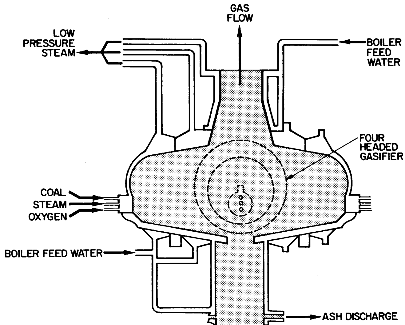
Figure 1. Koppers-Totzek gasifier.
