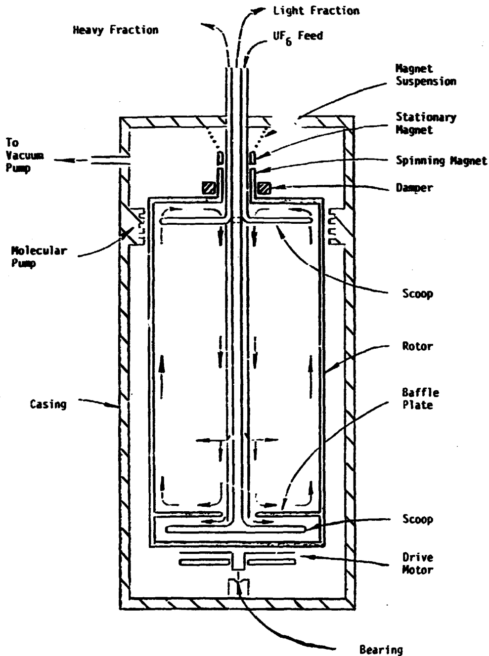
Fig. A-1. ZIPPE Centrifuge (Simplified).
