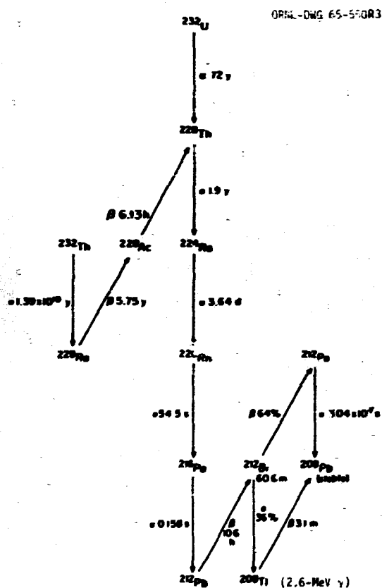
Fig. 3.0-1. Decay of ^{232}\text{U} .
