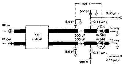
Fig. 6. 180^\circ phase shifter module.
