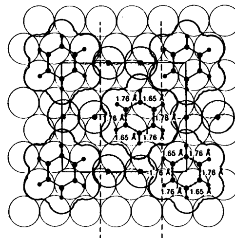
Pt(111) - (2√3×4)rect - 2C 6 H 6 + 4CO
