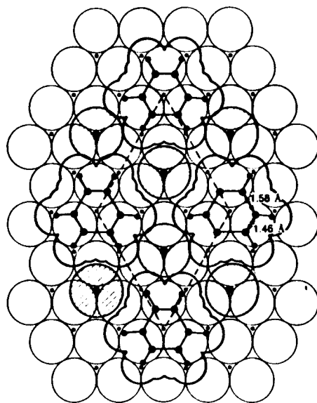
Rh(111) - (3×3) - C 6 H 6 + 2CO
