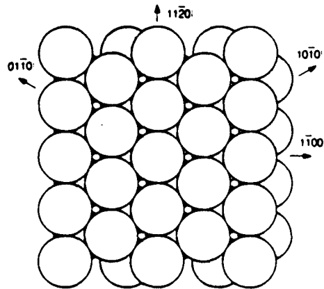
hcp (0001)
