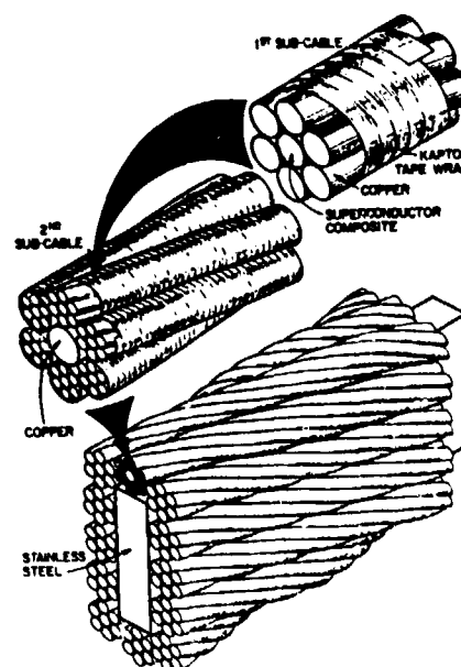
Fig. 5. - Superconductor cable composite
