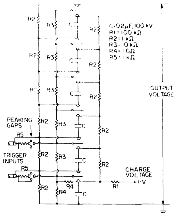
Fig. XVII-22. HDZP Marx module circuit diagram.
