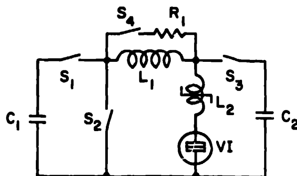
Fig. 1. Test circuit.
