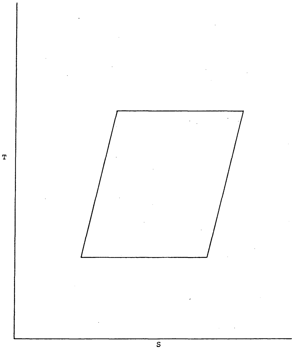
Fig. 4.1.2.2-1 Carnot-equivalent cycle
