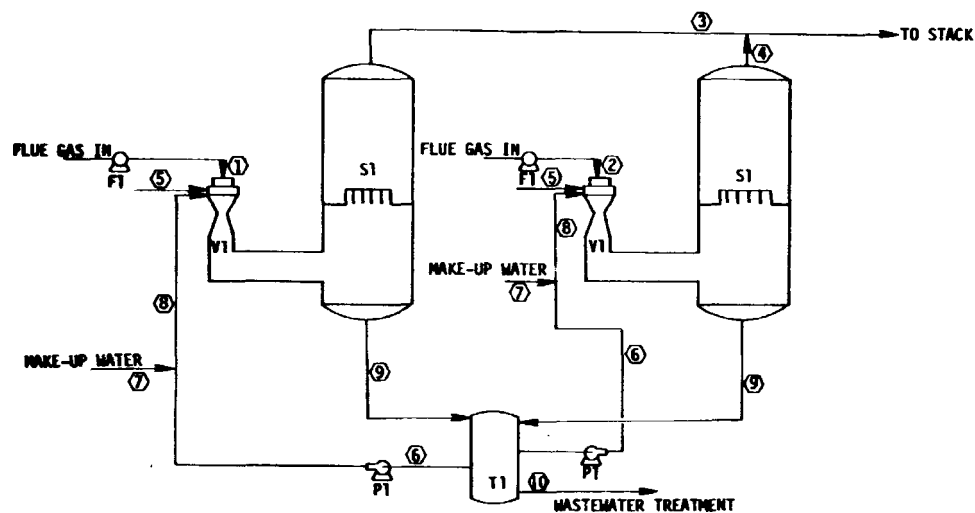
Figure 14-21. ITT Rayonier, Inc. Fernandina Beach, Florida.
