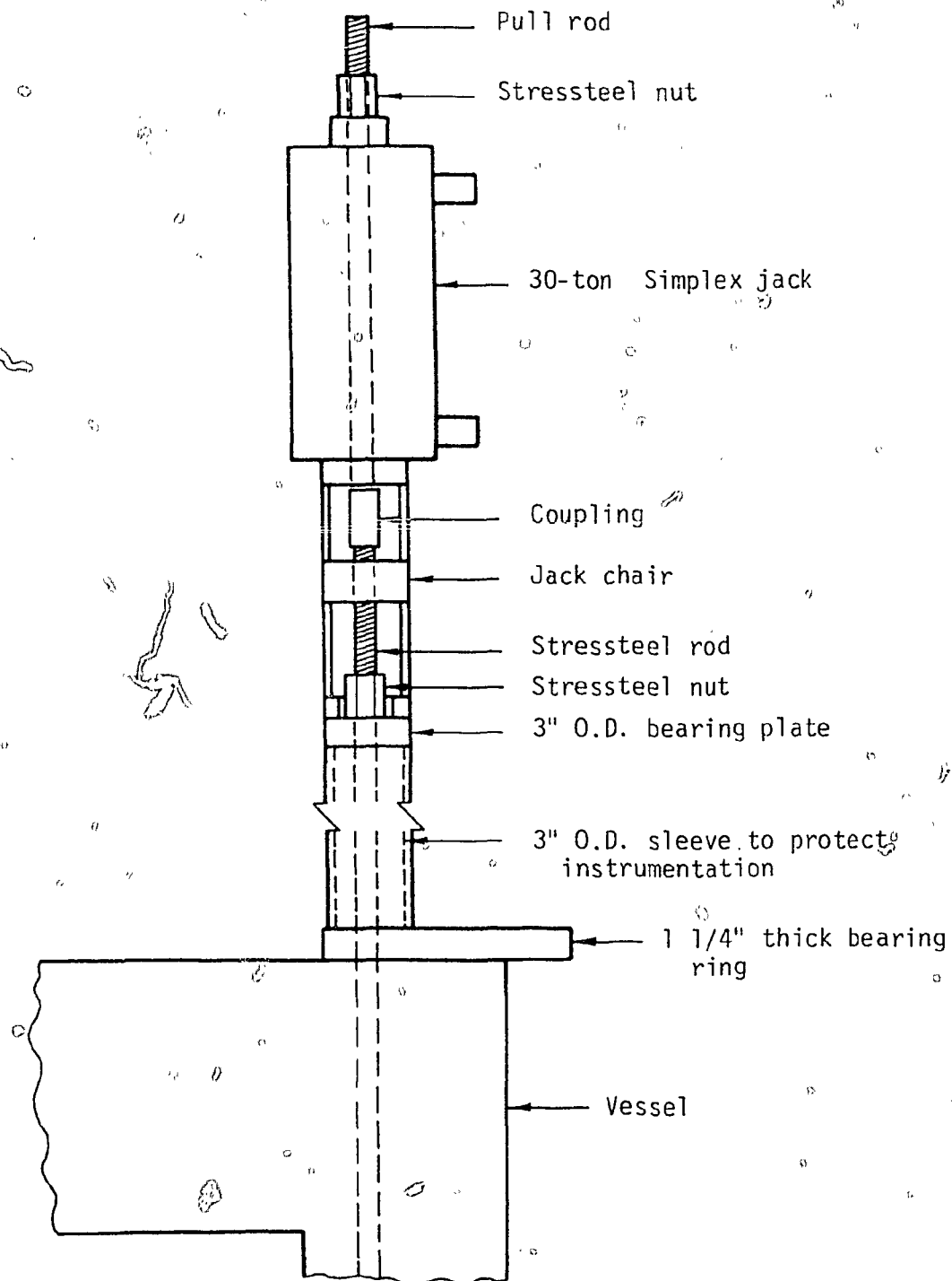
Fig. A.5 Apparatus Used for Longitudinal Prestressing
