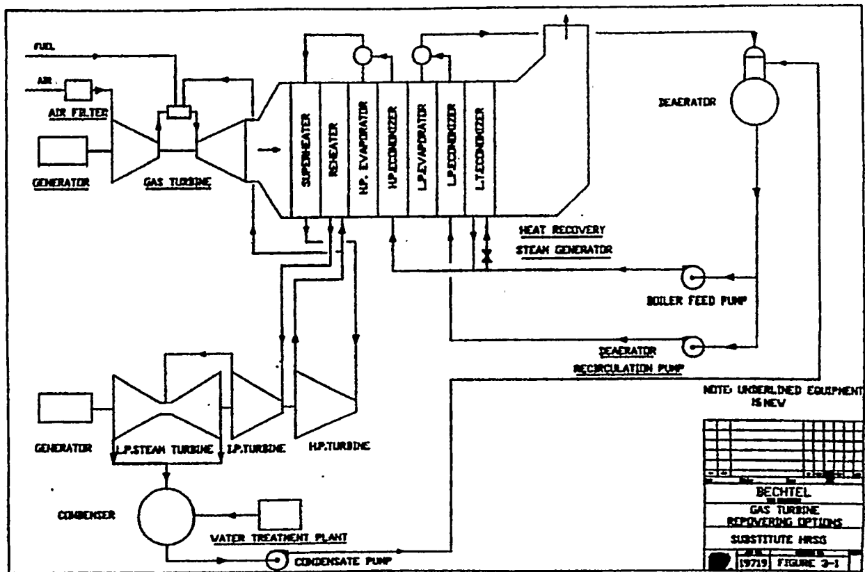
Figure 3.13-1 HRSG Substitution.
