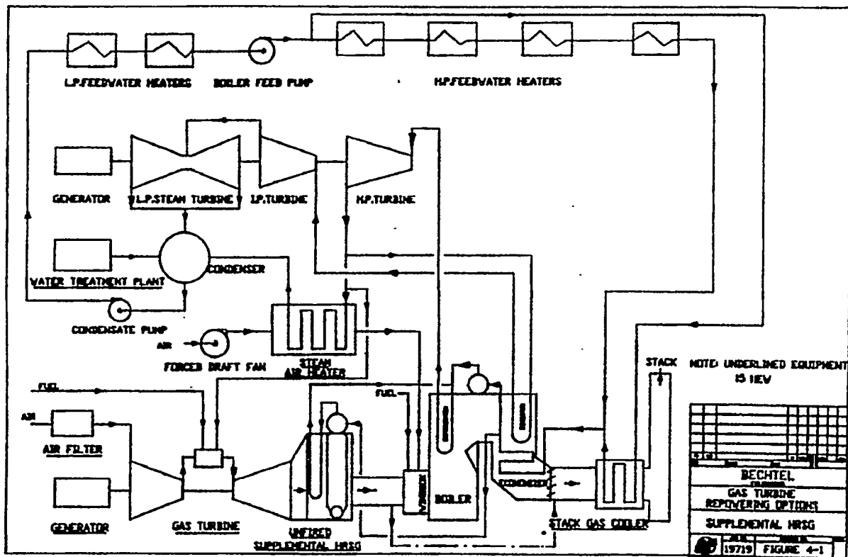
Figure 3.13-2 Supplemental HRSG.
