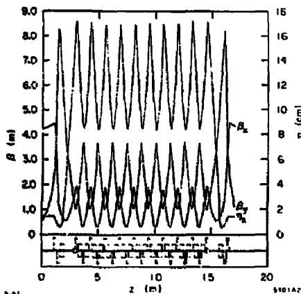
Fig. 2. Damping ring Twiss parameter display.
