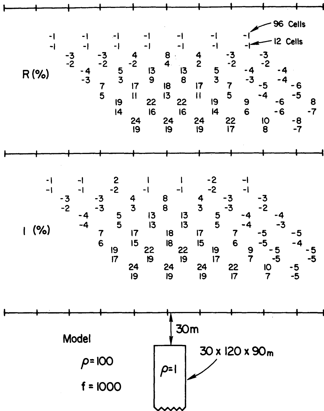
Figure 7 Convergence for Horizontal Loop EM
