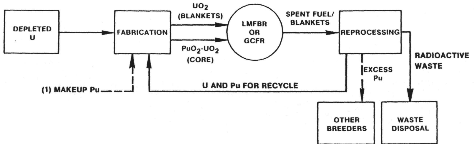
(A) URANIUM BLANKETS (LMFBR-Pu/U/U/U-HT OR GCFR-Pu/U/U/U)
