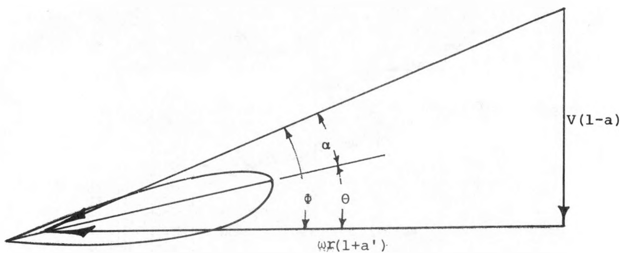
(b) Blade angles
