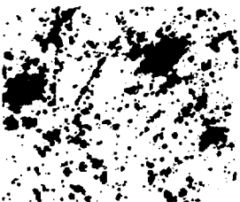
C-jet 4 c.u. Emulsion
