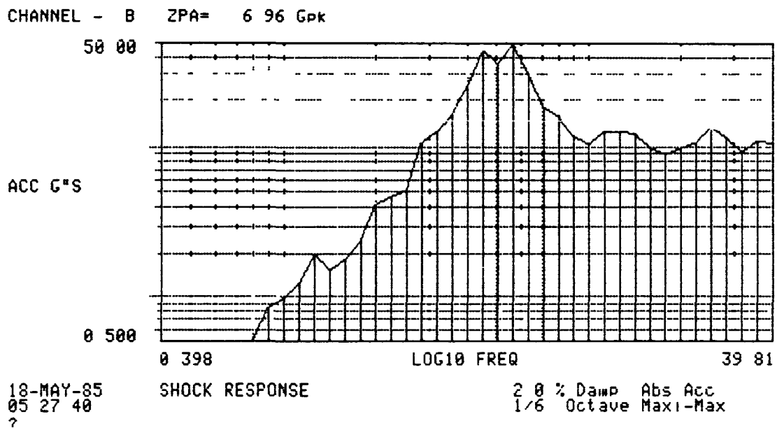
Figure 7 Actual Signal
