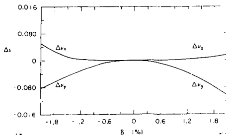
Fig. 1. Tune shift vs momentum
