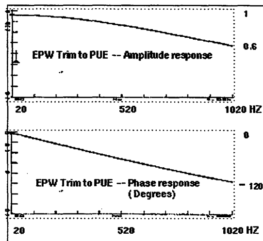
Figure 4: EPW trims to pues response.
