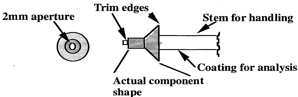
Fig. 3. Hohlraum mandrel design.
