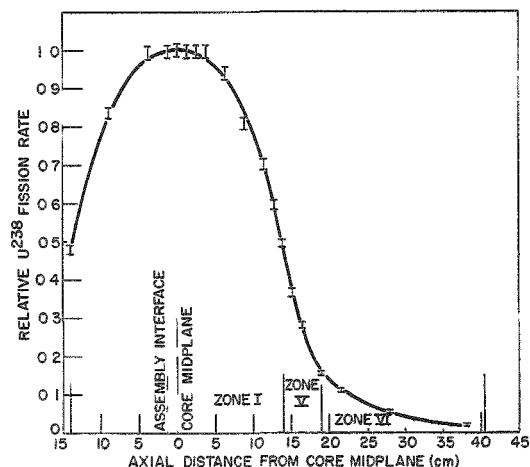
Fig. 21. U^{238} Axial Fission Traverse
