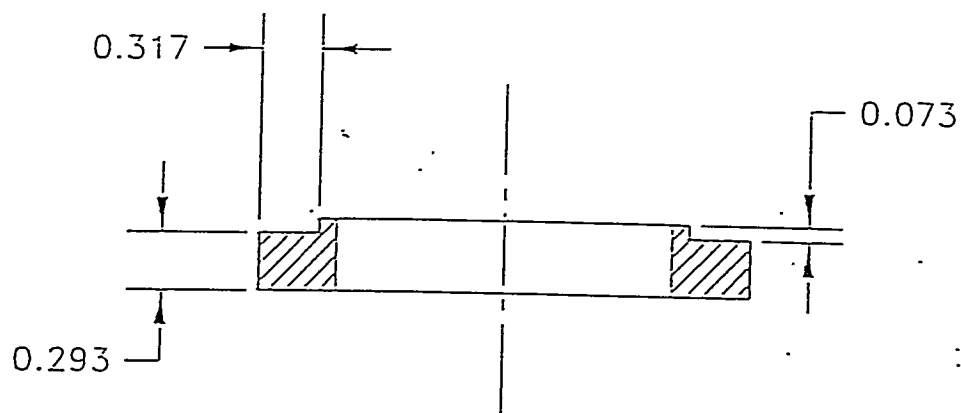
View A-A
