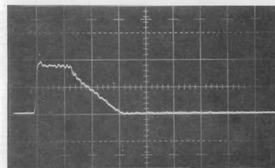
(d) Clock A3U, 2 V/cm 0.1 \mu sec/cm
