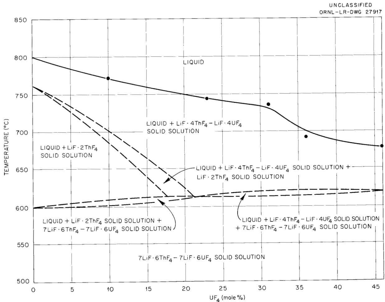
Fig. 2.3.8. The Join 7\text{LiF} \cdot 6\text{ThF}_4 - 7\text{LiF} \cdot 6\text{UF}_4 .
