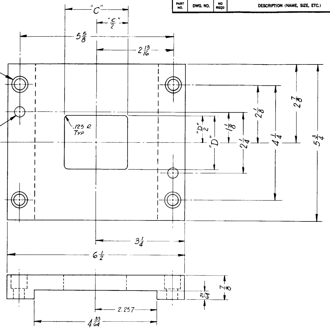
⑤ GUIDE PLATE MATL: Mild Steel 1 REQD
