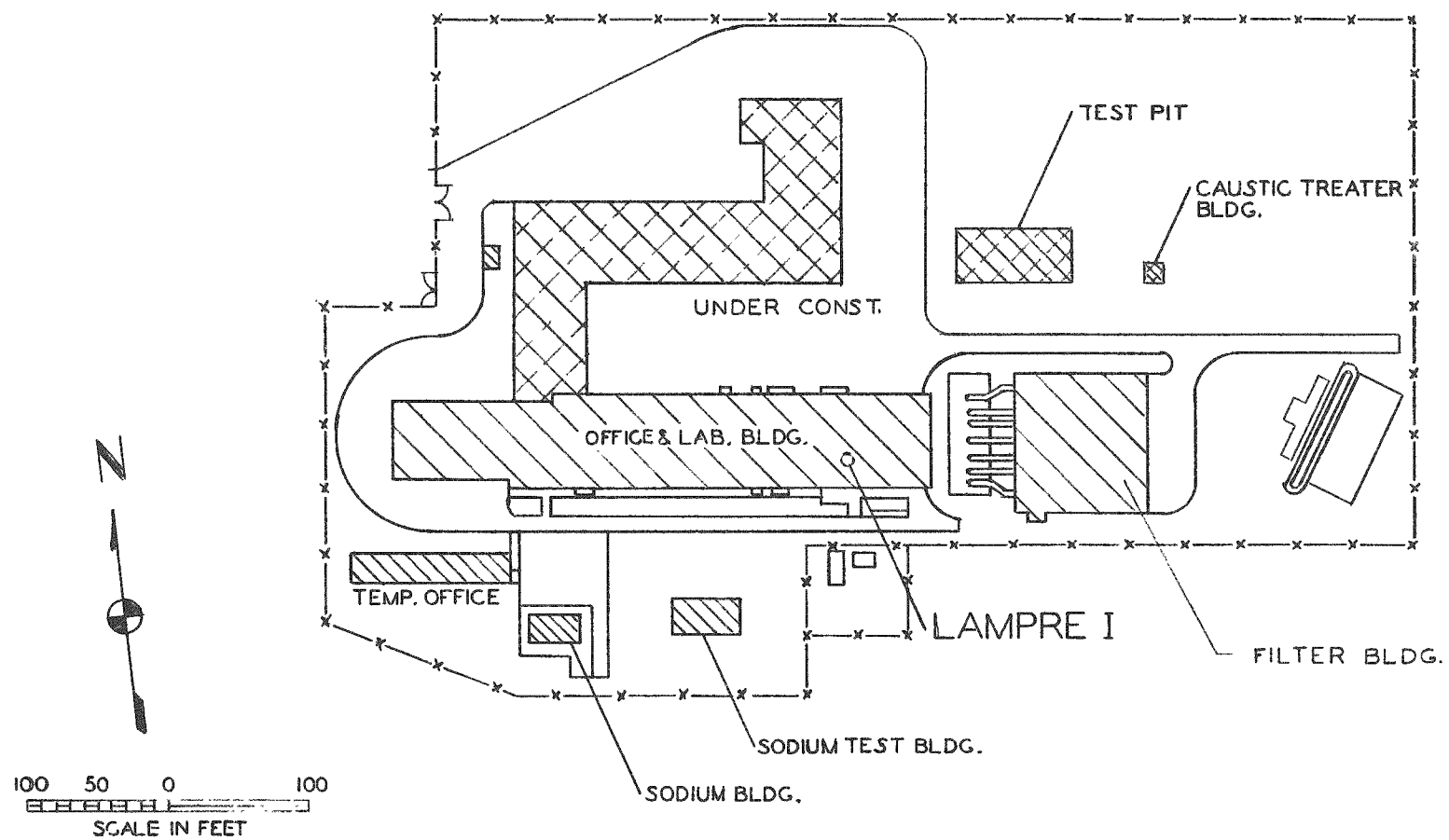
Fig. 3.4 Site layout.
