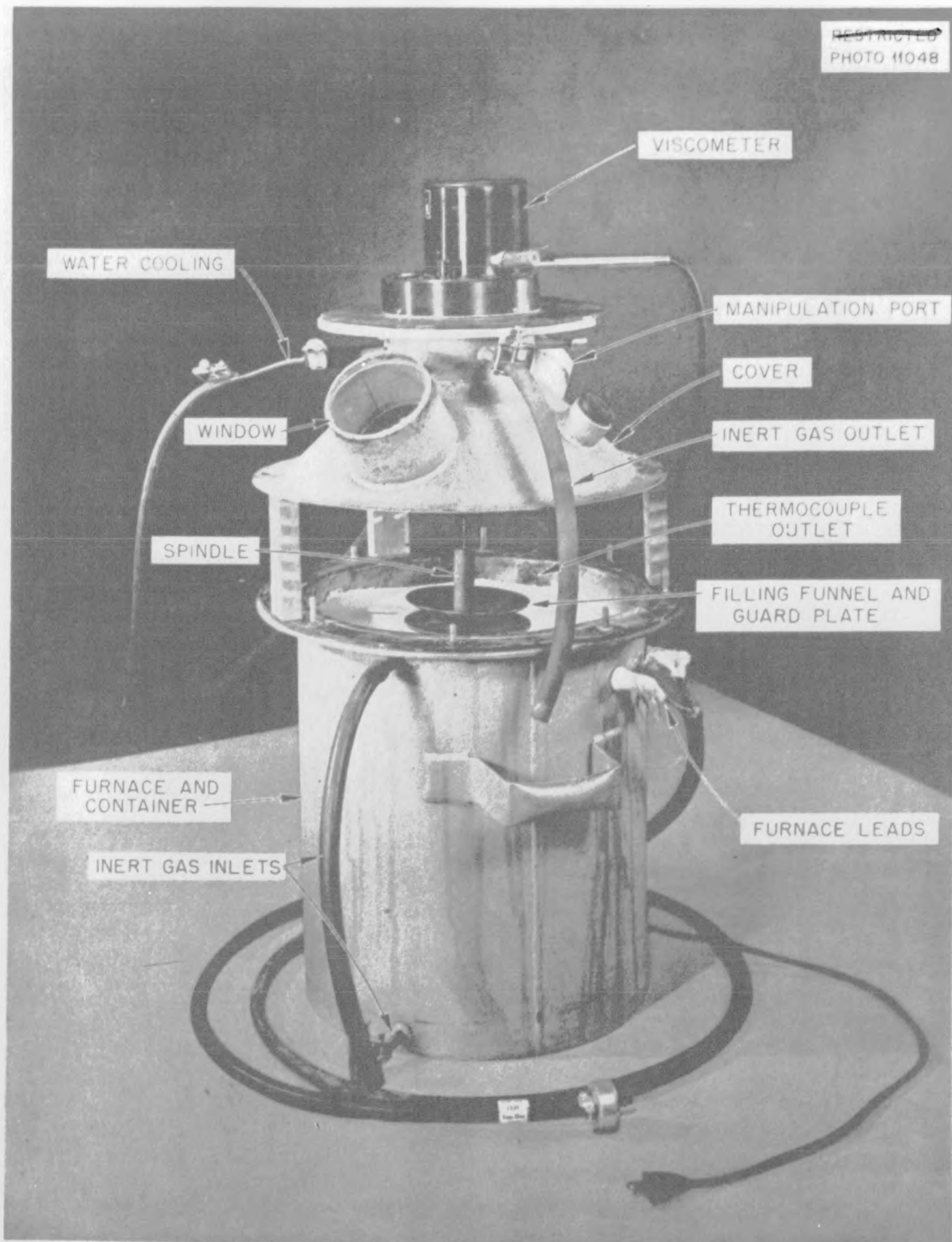
Fig. 12.4. Viscosity Apparatus.
