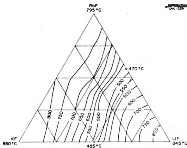
Fig. 10.5. The System KF-LiF-RbF.
