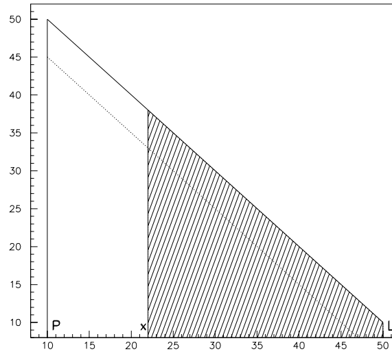
Sample Em 2x1 Distribution
