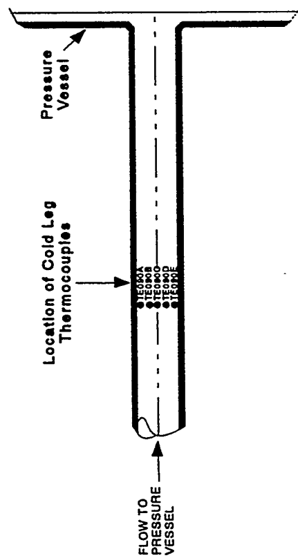
A-Loop Cold Leg
