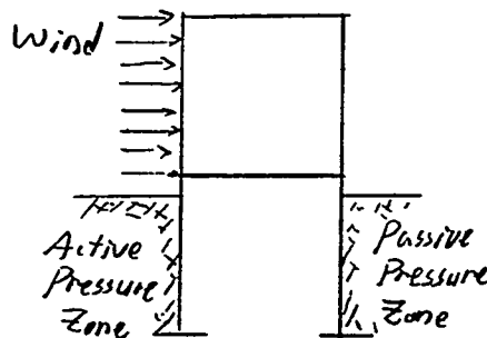
Superstructure Plus Basement
