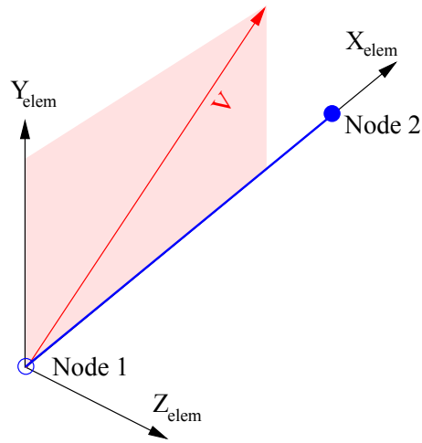
Input 5.12. Sierra/SD Mount Interface
