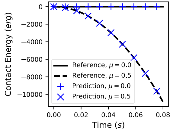
(d) Contact energy on a BT Shell inclined surface
