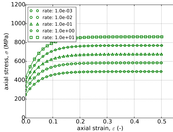
(c) Voce Hardening
