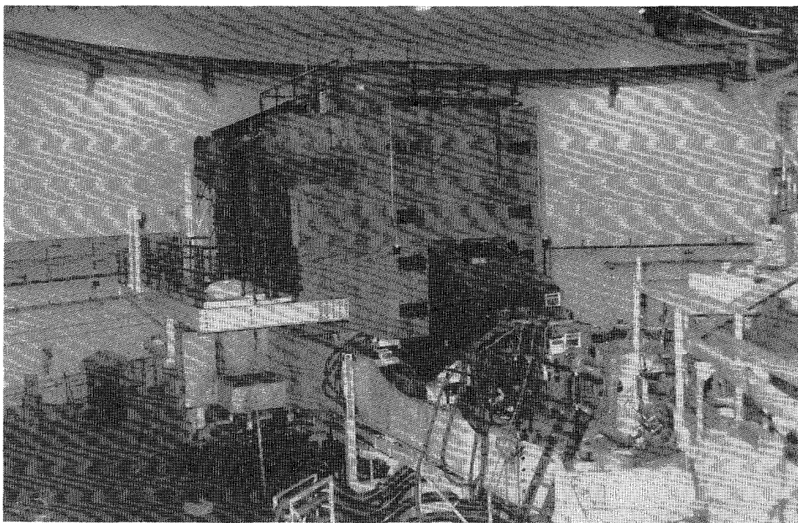
Fig. III-7. The HERMES spectrometer.
