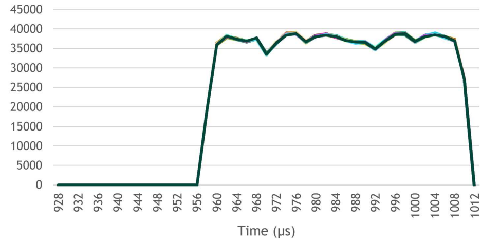
L2$ Hits
