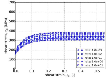
(i) Voce Hardening – 31
