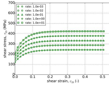
(h) Voce Hardening – 23
