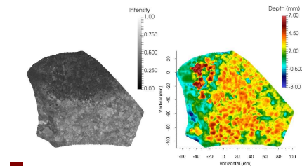
Asphalt
