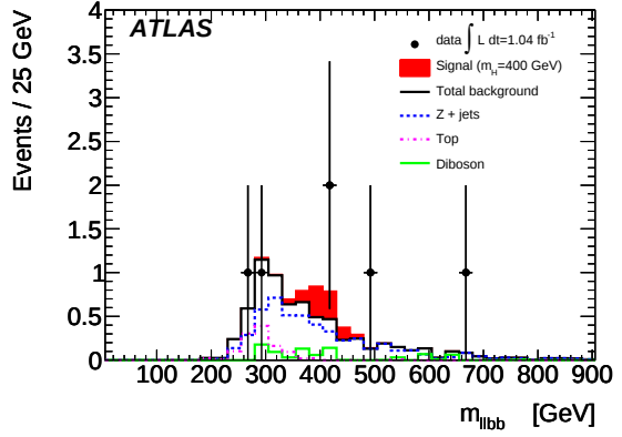
(d) High- m_H , tagged selection.
