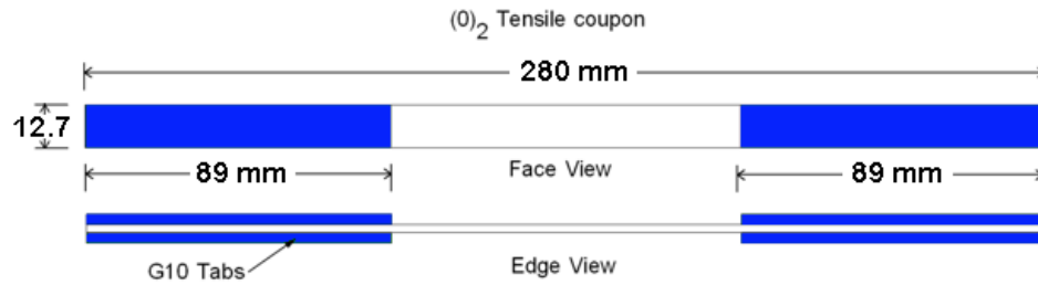
Longitudinal Tensile Coupon
