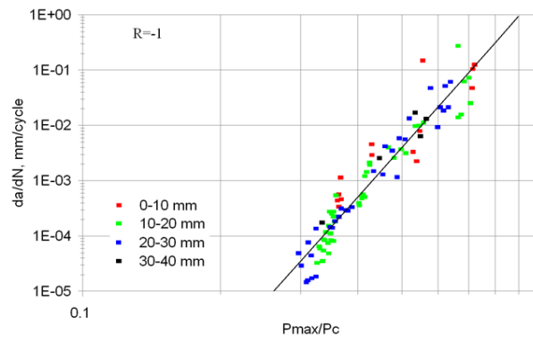
(d) Short CLS, no steel, R = -1
