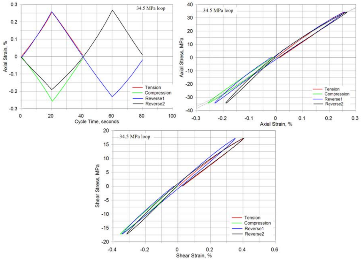
Figure35(d). 34.5 MPa
