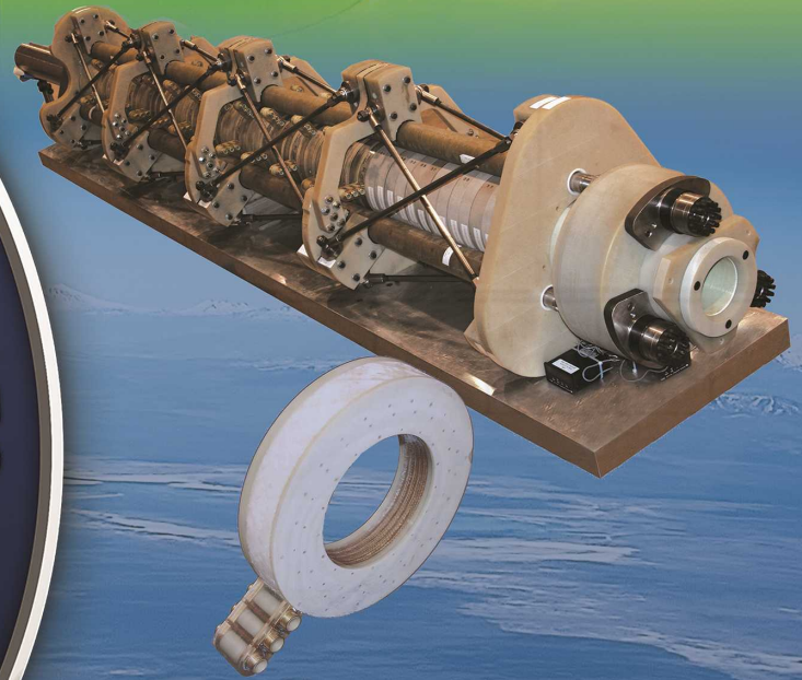
Navy EM Railgun
